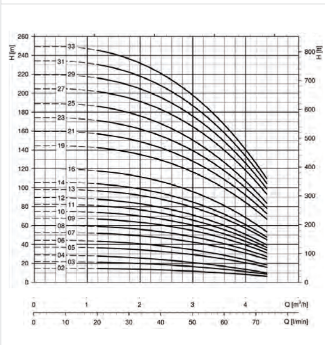
↳ 3SV
