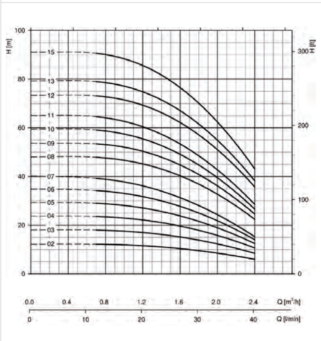
↳ 1SV : 2-15 stages
